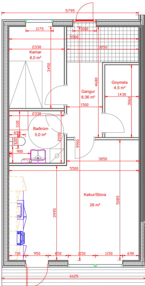
Tekning Heiðatrøðin 8A, D og G
