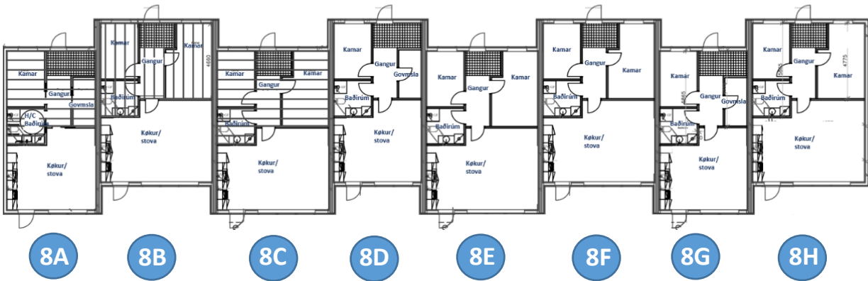
Tekning Heiðatrøðin 8A, D og G
