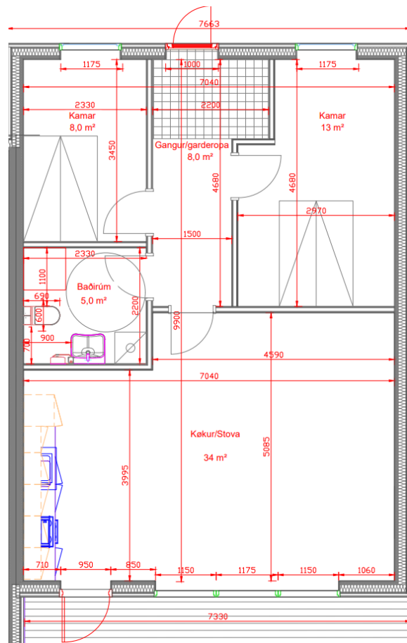
Tekning Heiðatrøðin 8B, C, E, F og H
